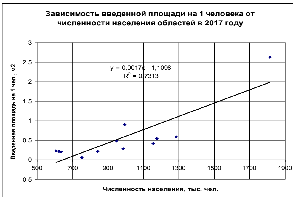
Рисунок 1 – Опытные данные и график регрессионной зависимости
